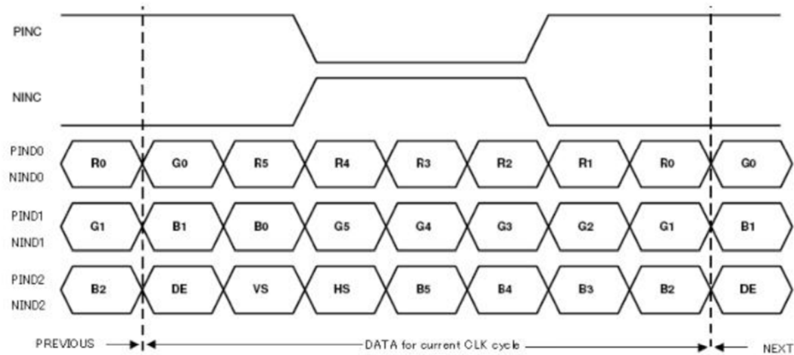
6bits LVDS Input
